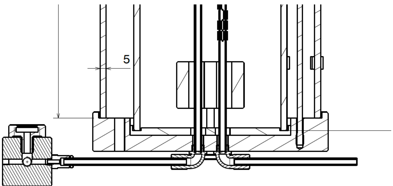
Abbildung 3: Ausschnitt des in [7] beschriebenen Borosilikatboilers, Tobias Tritschler Dipl.-Ing. Armin Rohnen LbA Fakultät 03 Labor für Schwingungstechnik und Maschinendynamik
